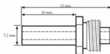
Långt munstycke
