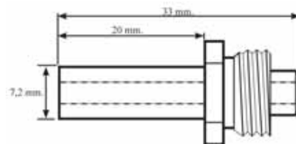
Långt munstycke
