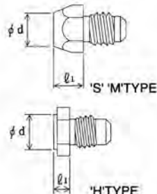
AR-2000MV
